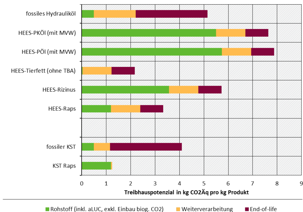
Abbildung 4-5 Treibhauspotenzial durch ausgewählte Lebenswege von biobasierten Schmierstoffen und Hydraulikflüssigkeiten (oben mit aLUC, unten ohne aLUC)
