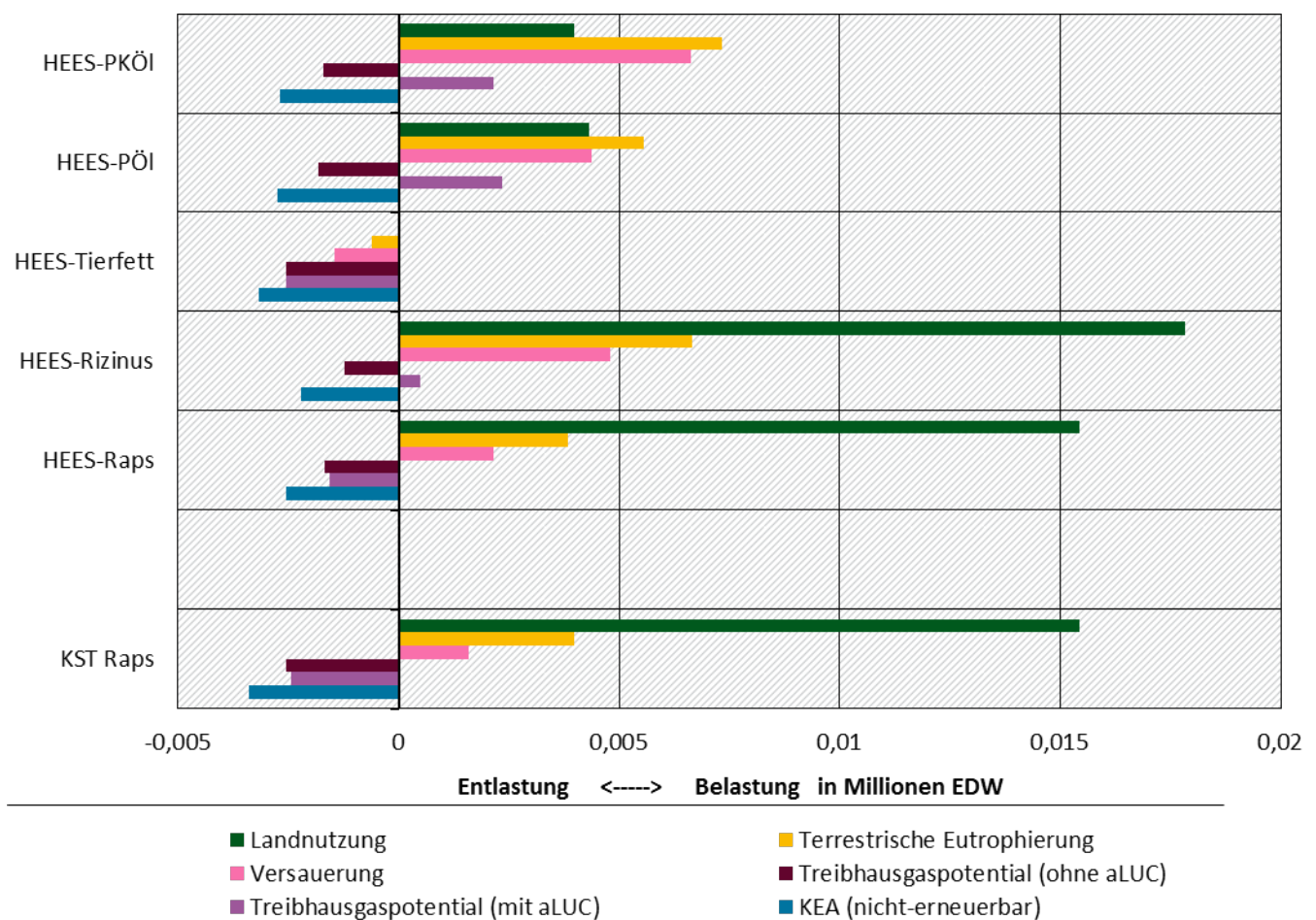
Abbildung 4-9 Normierung der Wirkungsabschätzungsergebnisse für biobasierte Schmierstoffe und Hydrauliköle
