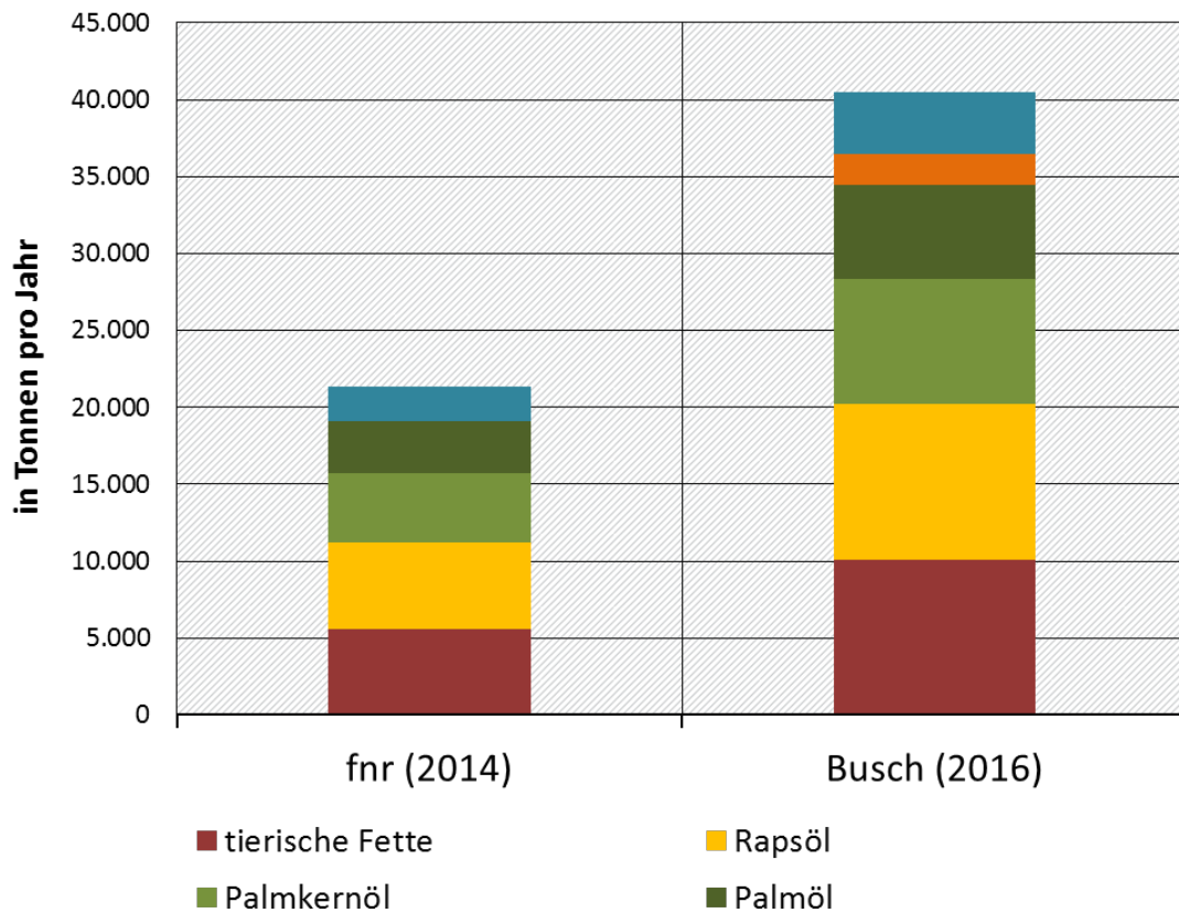
Abbildung 3-5 Einsatzmengen an Pflanzenölen und Tierfetten für die Herstellung von Bioschmierstoffen in Deutschland
