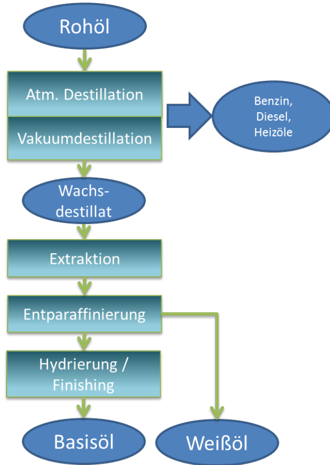
Abbildung 4-3 Prozessschritte der Grundölraffination (eigene Darstellung)
