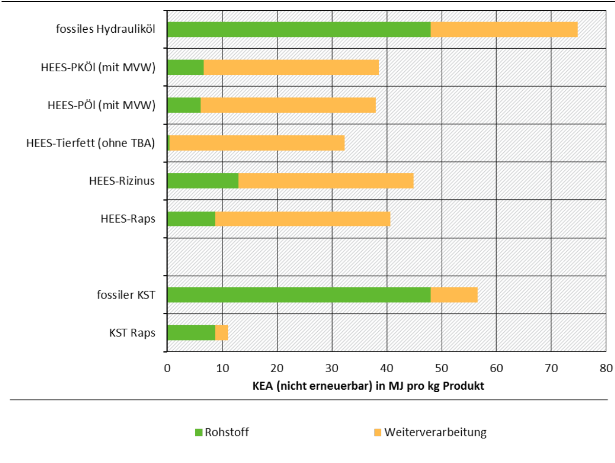
Abbildung 4-4 Kumulierter Primärenergiebedarf (KEA) durch ausgewählte Lebenswege von biobasierten Schmierstoffen und Hydraulikflüssigkeiten
