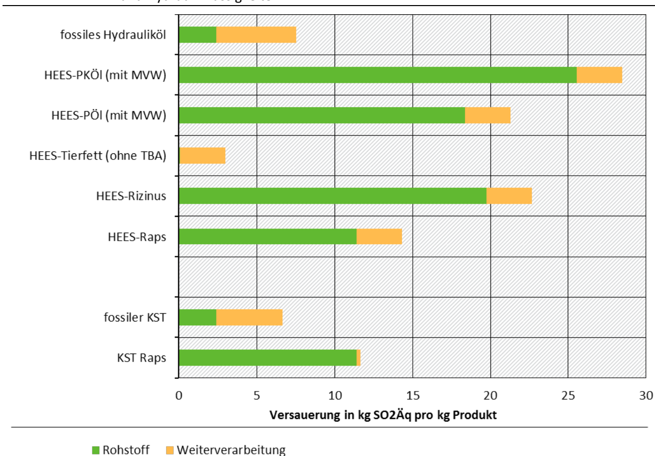
Abbildung 4-6 Versauerungspotenzial durch ausgewählte Lebenswege von biobasierten Schmierstoffen und Hydraulikflüssigkeiten
