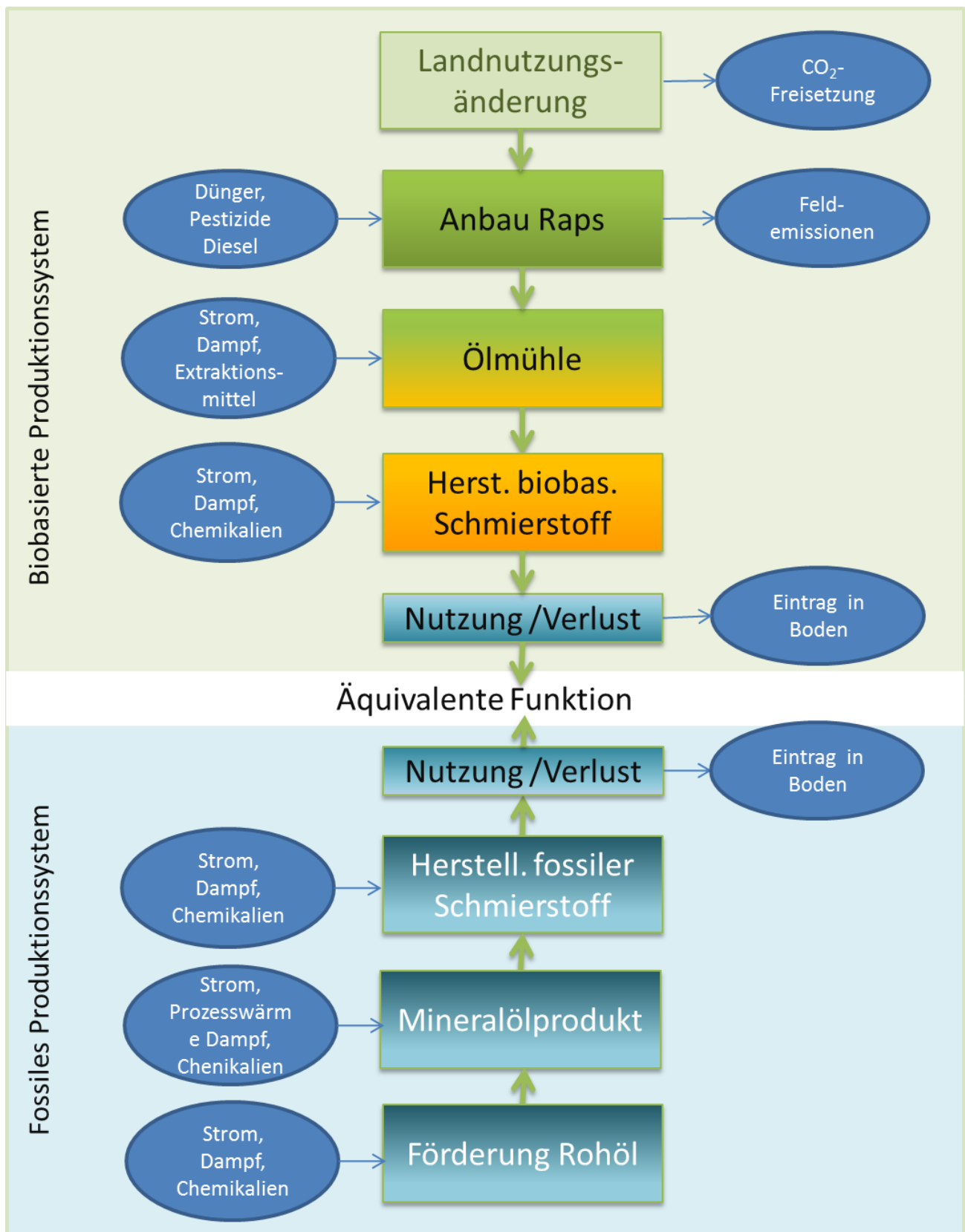
Abbildung 4-2 Systemgrenze der Übersichts-Ökobilanz für biobasierte Schmierstoffe und Hydraulikflüssigkeiten (Bsp. Rapsöl)
